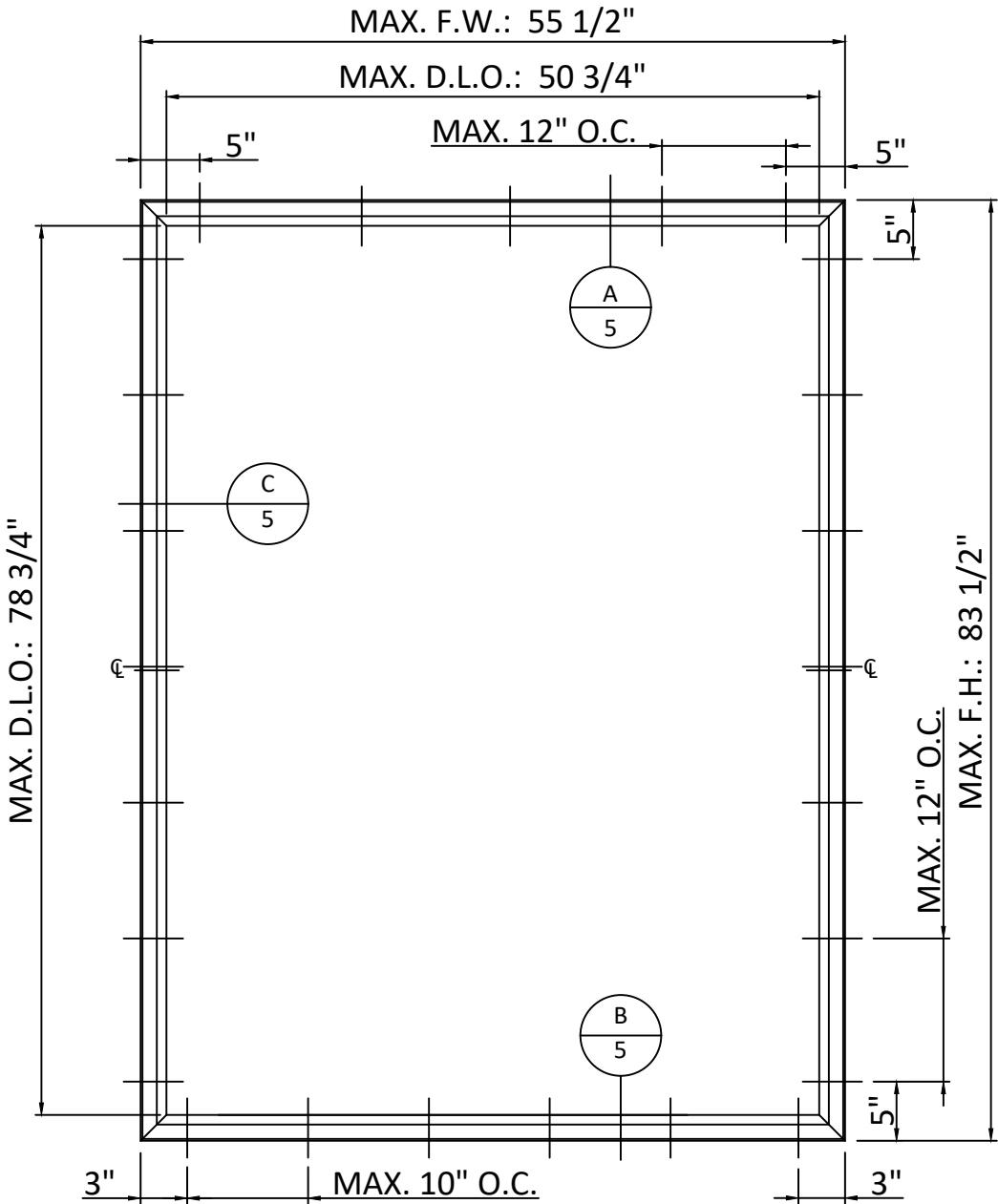
ELEVATION
